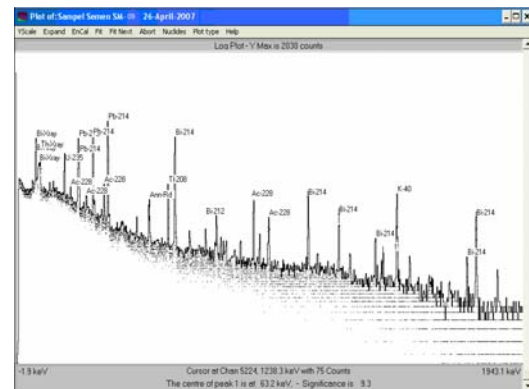
Gambar 4. Spektum sinar- \gamma cuplikan semen (kode cuplikan SM-09).
