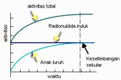
Gambar 2. Kesetimbangan sekular pada peluruhan nuklida umur panjang.
